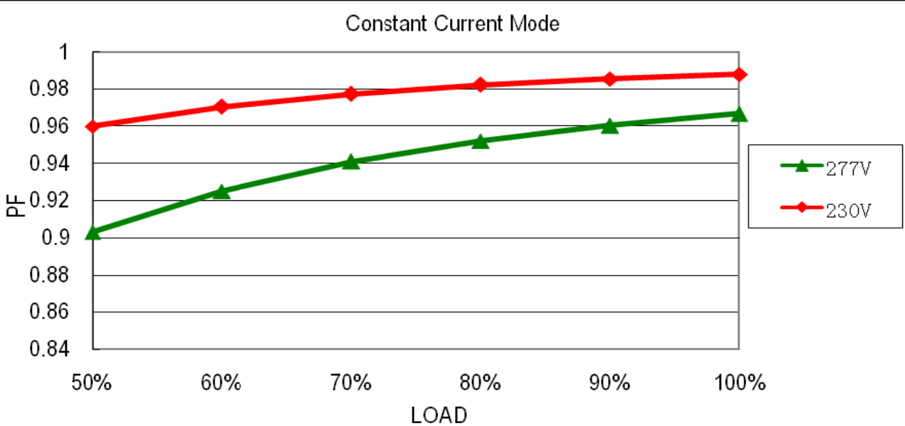
P.F vs LOAD
